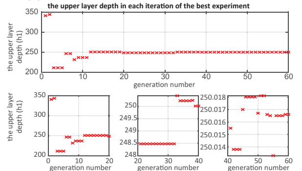
(D) The upper layer depth in the best experiment
